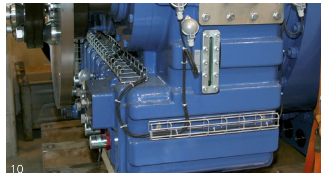
Abb. 7: Gitterkanal zur Kabelführung im Turm Fig. 7: Wire tray to the cable routing in the tower
